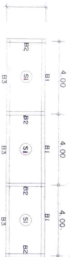
แปลนถนน, หนา คัด คสส. 1:100
